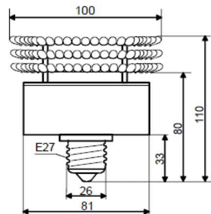
Obelux 32-48-E27
